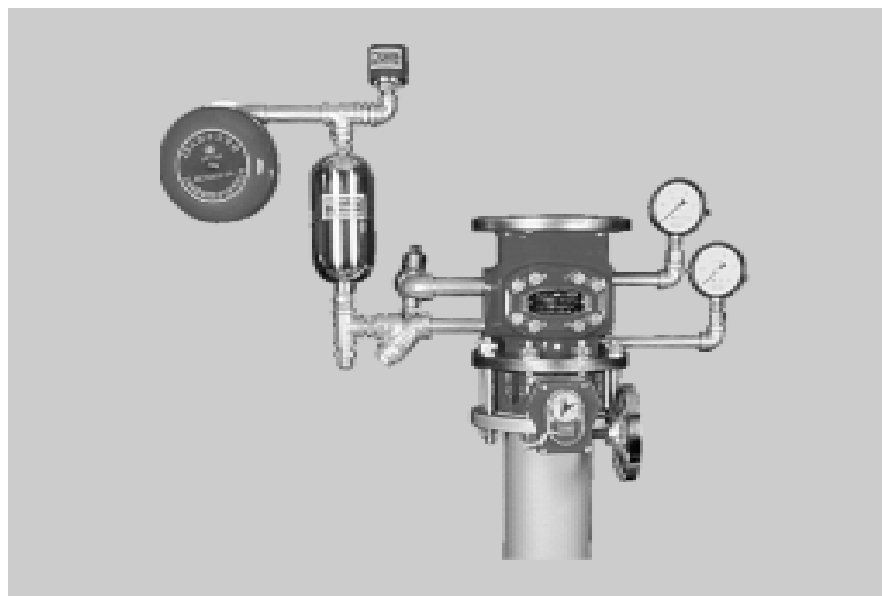
ZSFZ 型湿式报警阀装置
